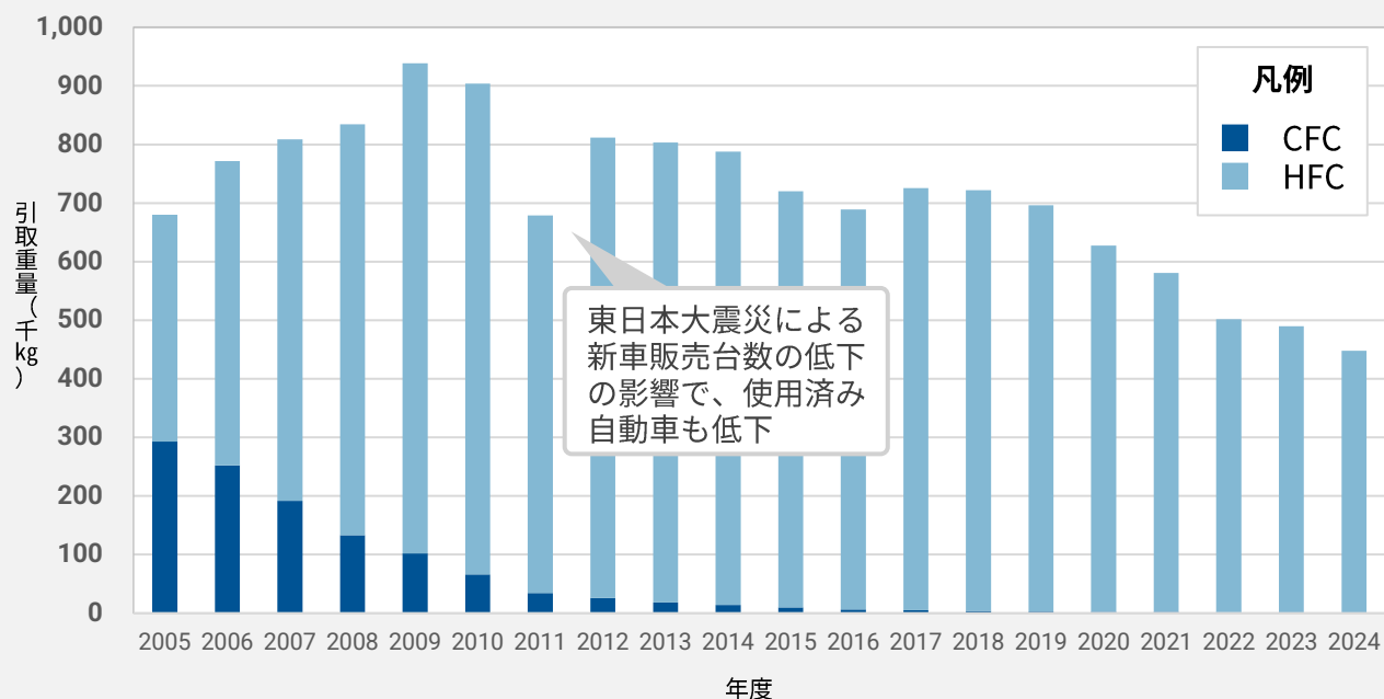
図2 フロン種別別フロン引取量の推移 (2005-2024)
