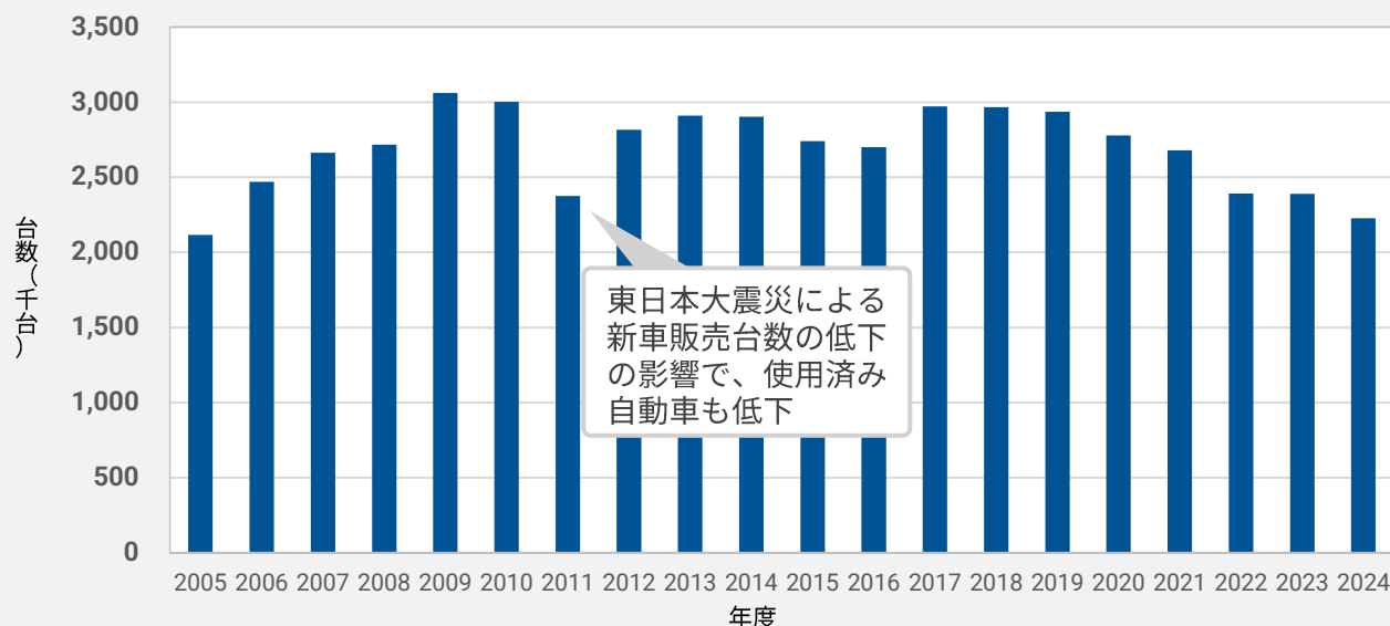
図1 フロン引取台数の推移 (2005-2024)
